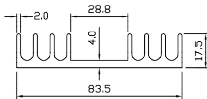
SP 5109 WT – 1.548 KG/M PERIMETER – 367.523 MM
