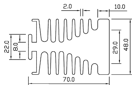
SP 5051 WT – 5.449 KG/M PERIMETER – 679.709 MM
