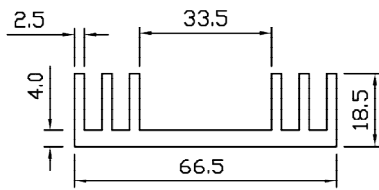
SP 5024 WT – 1.305 KG/M PERIMETER – 315.00 MM
