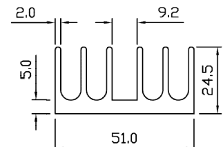
SP 5107 WT – 1.378 KG/M PERIMETER – 328.059 MM
