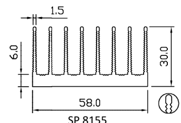
SP 8155 WT – 1.650 KG/M PERIMETER – 603.055 MM
