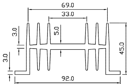
SP 5006 WT – 2.500 KG/M PERIMETER – 632.982 MM
