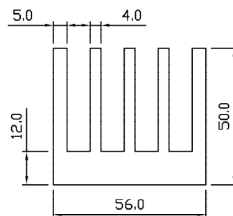
SP 0189 WT – 4.072 KG/M PERIMETER – 516.000 MM
