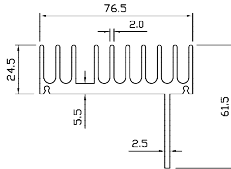
SP 5106 WT – 2.434 KG/M PERIMETER – 603.578 MM
